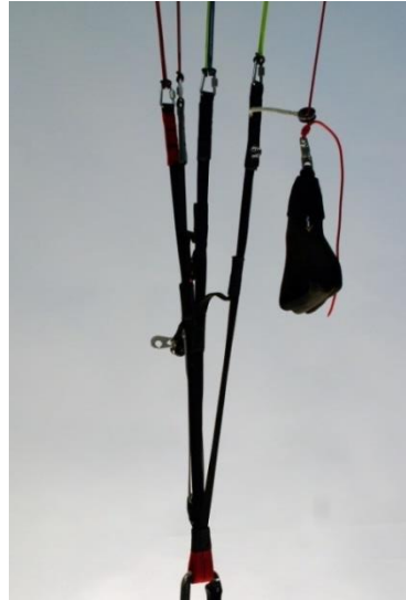
Fig. 3 ARCUS RS riser
